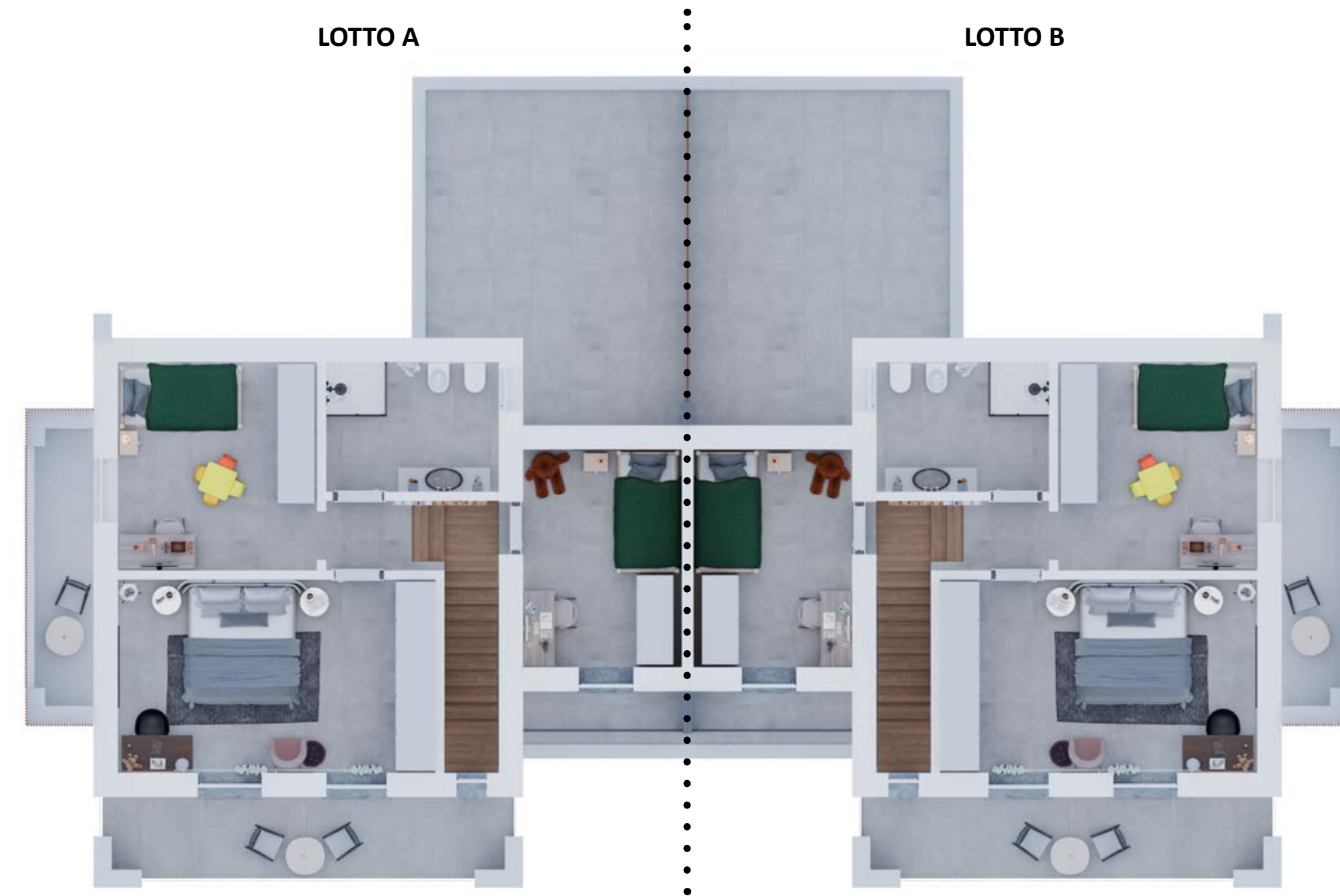
Planimetra generale primo piano
